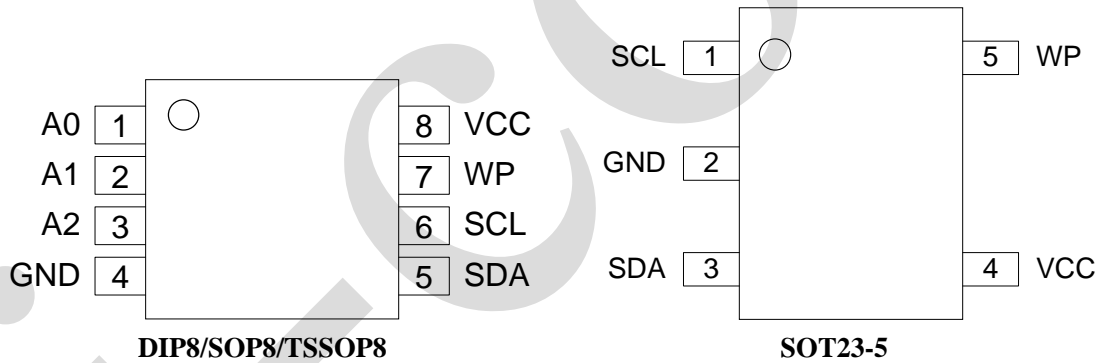
图 2、引脚排列图
